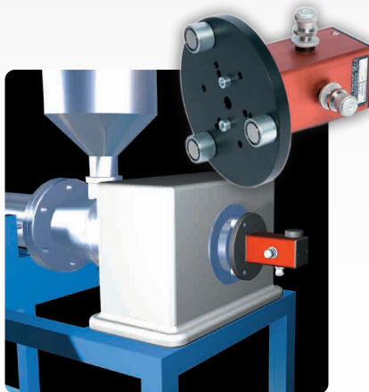
Trasmittitore laser sul mandrino della scatola del cambio.
